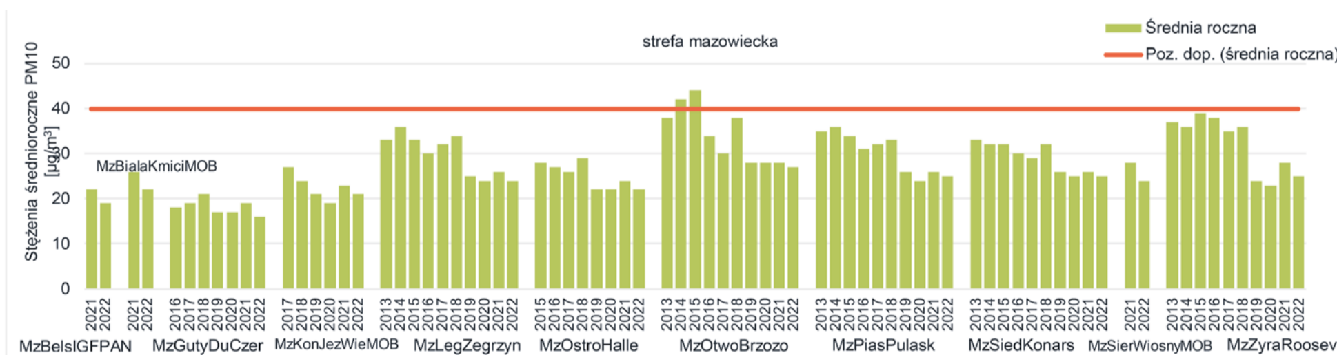
Rysunek 7.28. Przebieg wartości średniej rocznej stężenia pyłu zawieszonego PM10 na poszczególnych stanowiskach pomiarowych w województwie mazowieckim na tle poziomu dopuszczalnego w latach 2013 - 2022 [źródło: GIOŚ]
