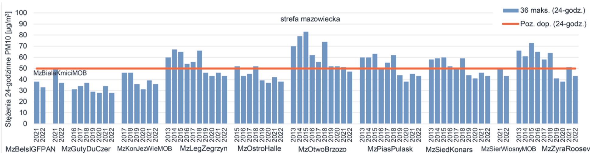
Rysunek 7.27. Przebieg 36 maksymalnej wartości 24-godzinowej stężenia pyłu zawieszonego PM10 na poszczególnych stanowiskach pomiarowych województwa mazowieckiego na tle poziomu dopuszczalnego w latach 2013 - 2022 [źródło: GIOŚ]
